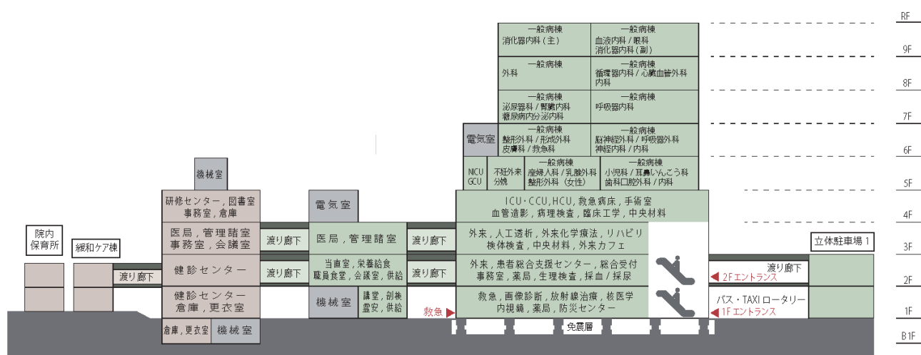
断面計画
